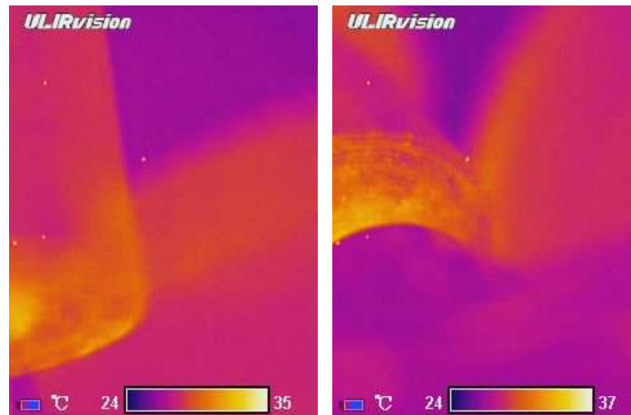
Рис. 11. Розподіл температури під час фрезерування розподільчого вала
