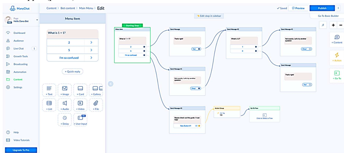
Рис. 4. Ієрархія повідомлень
