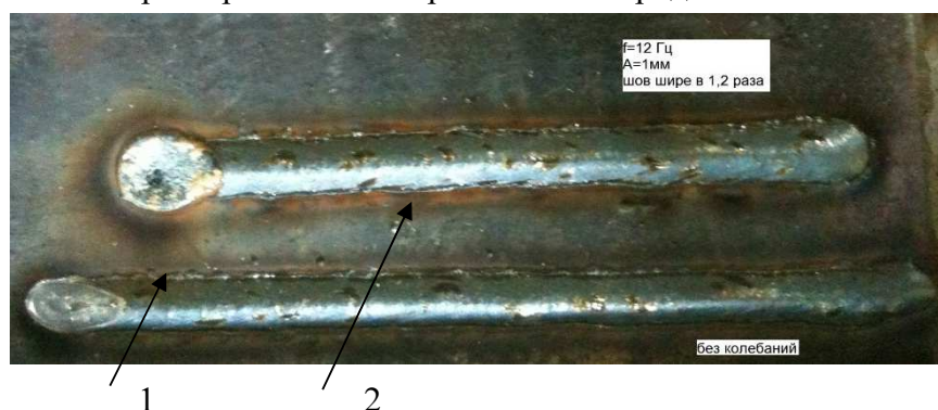
Рис. 2. Результаты сравнительной наплавки: 1 – без колебаний; 2 – с колебаниями
