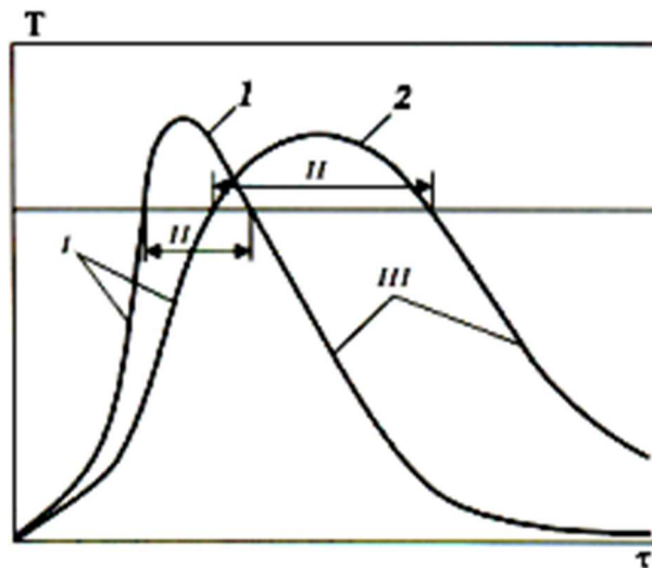
Рис. 2. Термічні цикли мікроплазмового (1) і аргонодугового (2) зварювання (паяння)
