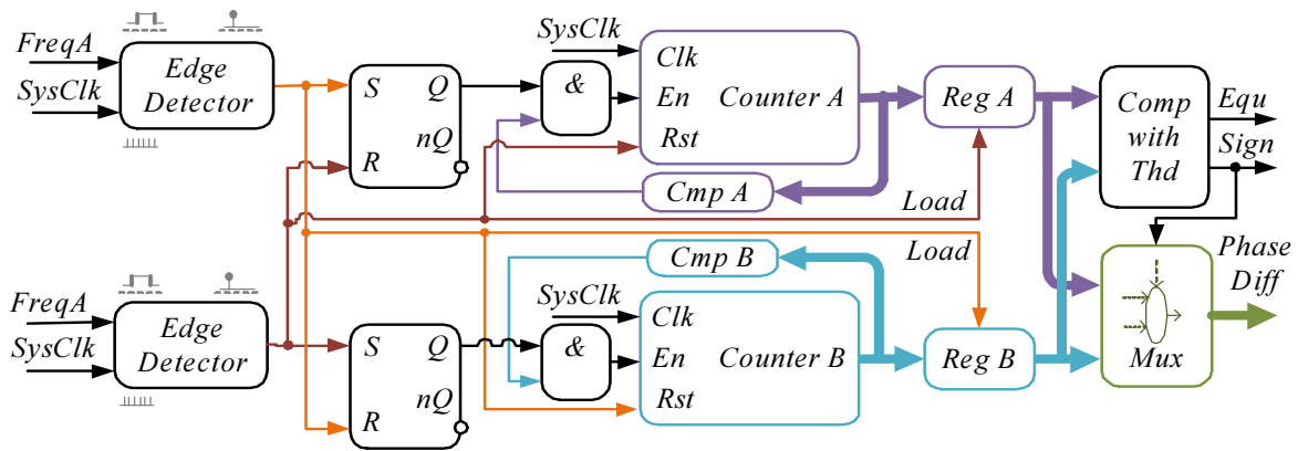
Рис. 5. Структурна схема блока ФК
