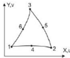
Рис. 3. Вузловий плоский скінченний елемент
